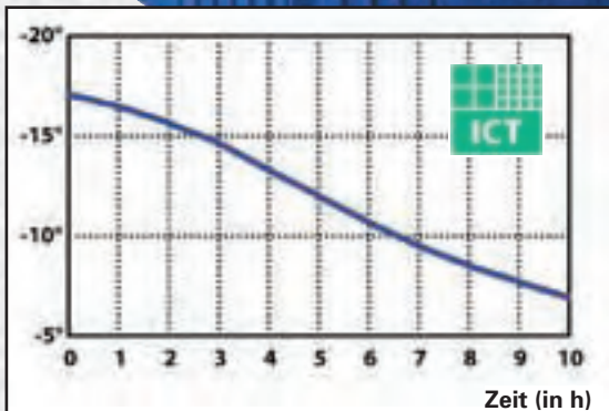
Temperaturverlauf Kühlhalten Thermo-Clipper Typ H1120 GN1/1 15 kg Tiefkühlgut ohne Kühlakkus Einfülltemperatur: -18°C Umgebungstemperatur: +20°C
